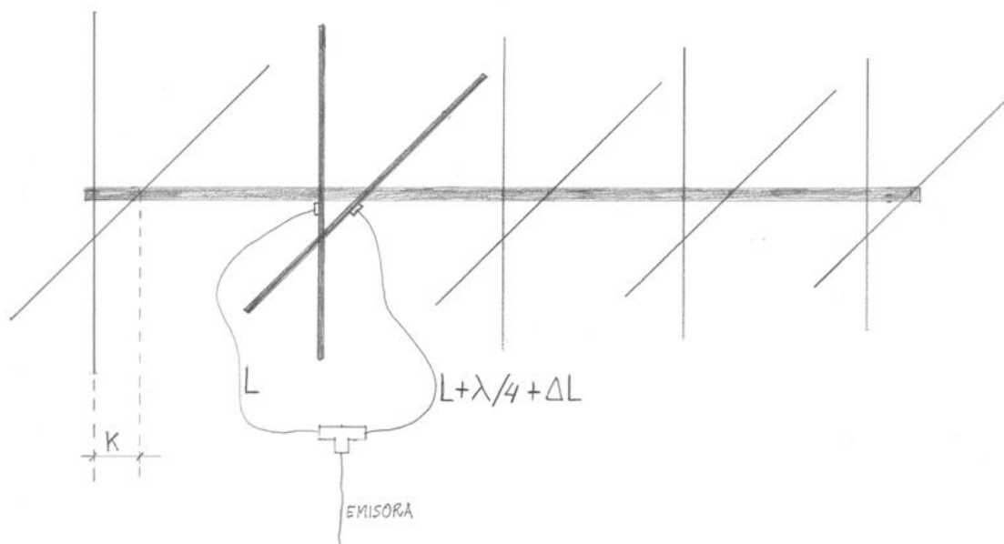
Figura n°3 Antenas desfasadas \frac{1}{4} \lambda mediante línea de alimentación teniendo en cuenta el desfase mecánico
