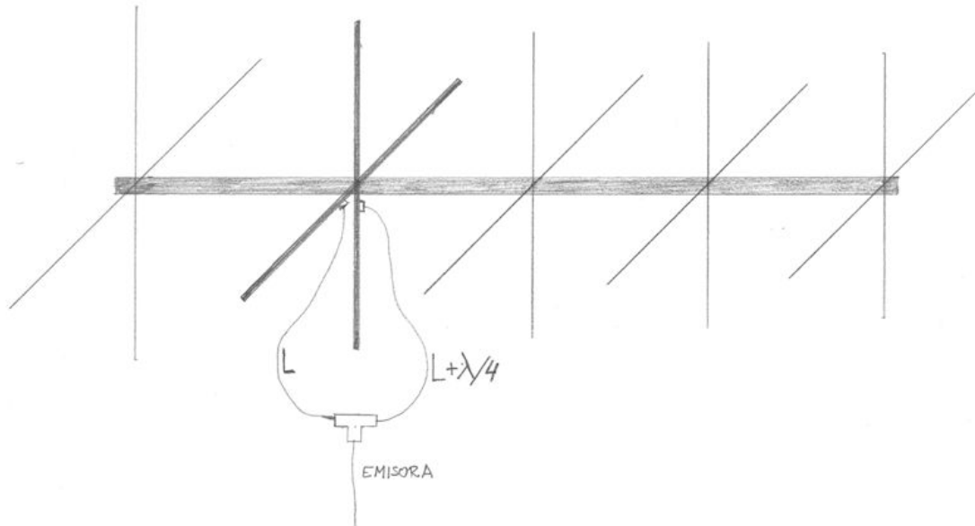
Figura n° 2 Antenas desfasadas \frac{1}{4} \lambda mediante línea de alimentación
